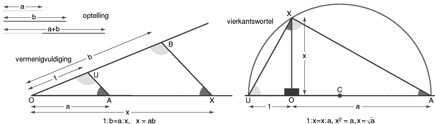
Figuur 4 Constructies met passer en liniaal. Euclidische constructies met passer en liniaal kunnen vijf arithmetische operaties geven: optellen, aftrekken, vermenigvuldigen, delen en worteltrekken. Optellen is gewoon het achter elkaar leggen van lijnstukken, aftrekken is het omgekeerde. Vermenigvuldigen houdt in dat gelijkvormige driehoeken gemaakt worden wiens zijden de verhoudingen 1 : b = a : x voorstellen, dus x is het product van a en b . Delen is weer het omgekeerde. Voor worteltrekken worden gelijkvormige driehoeken in een cirkel ingeschreven, met zijden met verhoudingen 1 : x = x : a , zodat x^2 = a en de lengte van het lijnstuk x is de wortel uit a . Alleen deze vijf operaties zijn mogelijk; het is onmogelijk om derdemachtswortels te trekken, wat van belang is bij het bewijzen dat trisectie onmogelijk is.
