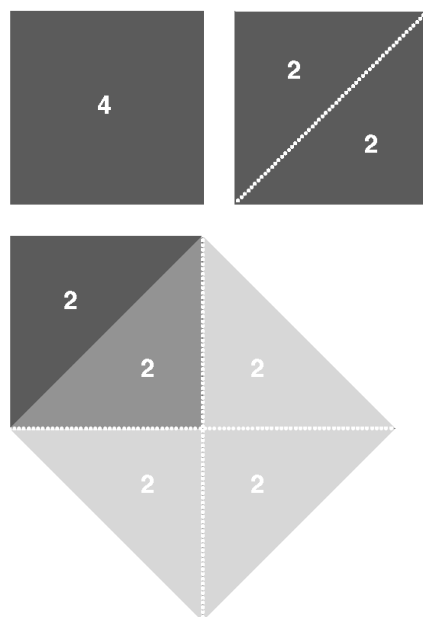
Figuur 2 Verdubbeling van het vierkant. Het verdubbelen van de vierkant is een bewijs dat aan een jongen slaaf werd geleerd in de Meno van Plato. Een vereenvoudigde versie begint met een vierkant met zijden 2 en oppervlakte 4, deelt deze langs de diagonaal, en maakt weer een nieuwe vierkant op die diagonaal. De gelijkbenige driehoek die de helft van het oppervlakte van het kleinere vierkant voorstelt is ook een kwart van het oppervlakte van het grotere vierkant, dus de oppervlakte is verdubbeld.
